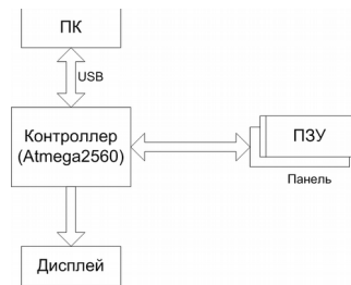
Рис.1 – Функциональная схема
