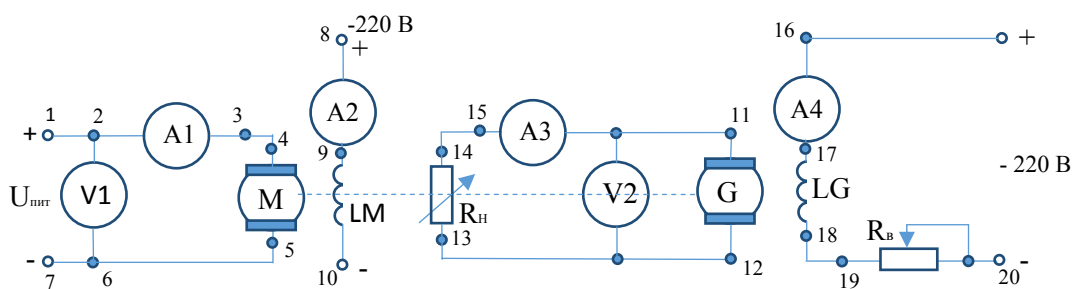
Рис.1. Электрическая цепь испытания двигателя постоянного тока параллельного возбуждения с нагрузочным генератором постоянного тока
